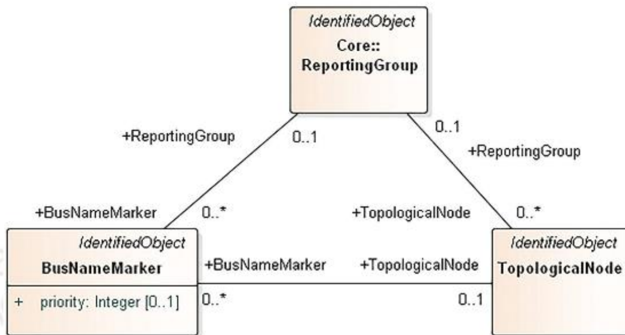
Рисунок А.2 — Диаграмма классов, описывающая группу объектов, используемую для построения отчетов
