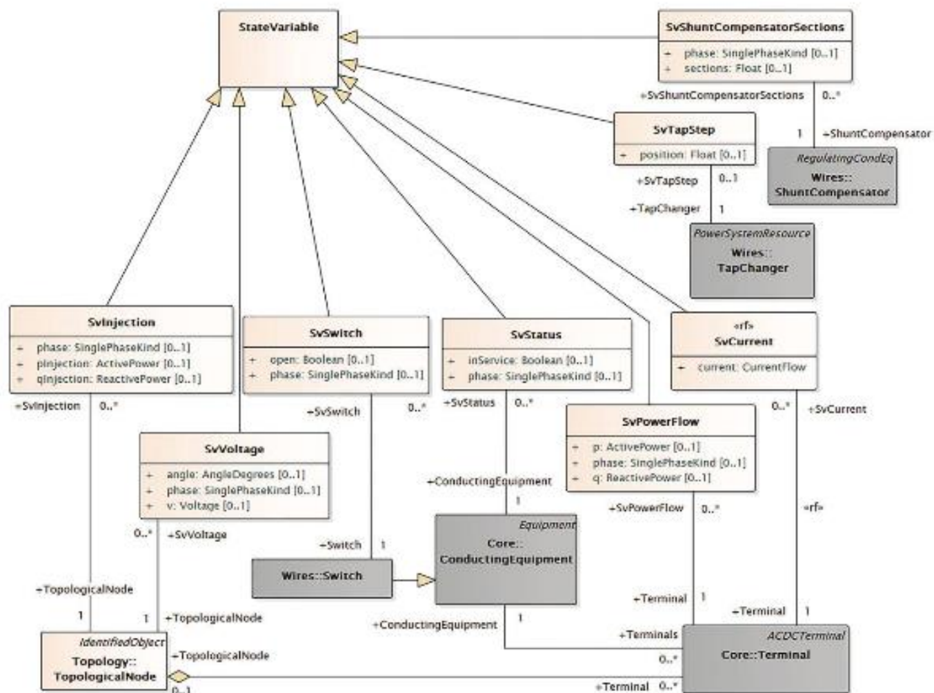
Рисунок А.8 — Диаграмма классов переменных состояния
