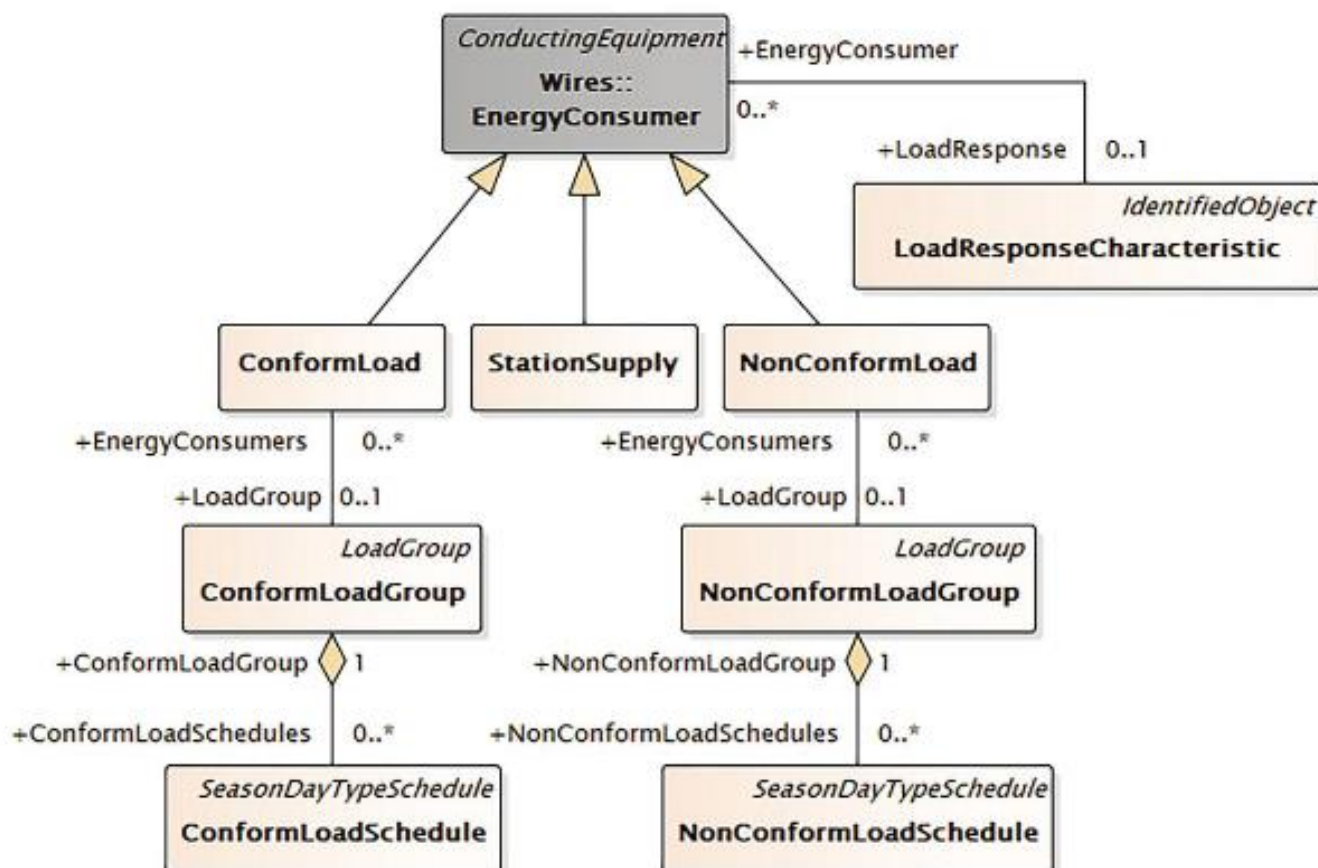
Рисунок А.3 — Диаграмма классов потребителей электрической энергии
