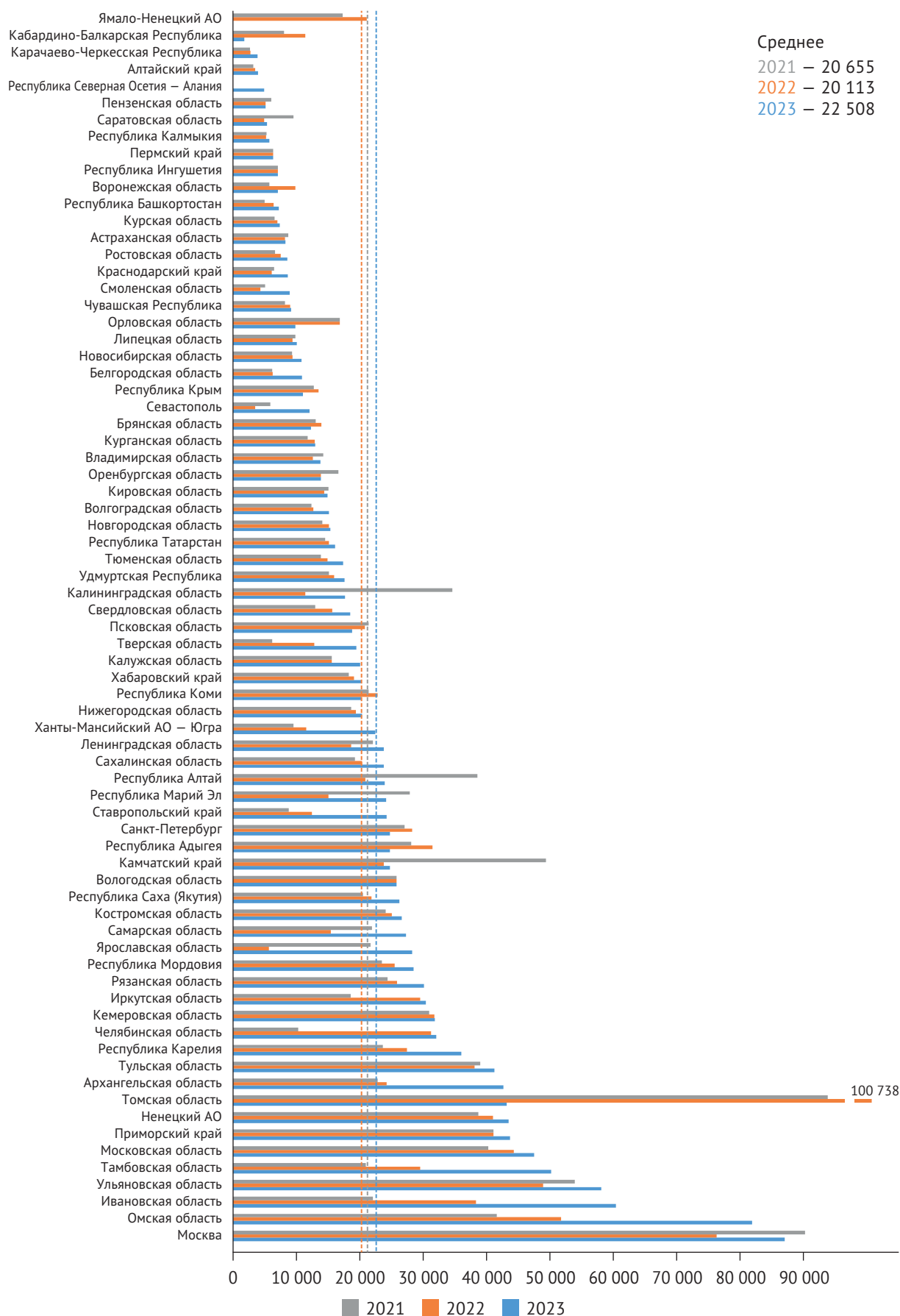
Рис. 33. Стандартизированная ставка на мониторинг выполнения заявителем ТУ и осуществление фактического присоединения (полиэтиленовый газопровод наружным диаметром 110–159 мм), руб./подключение
