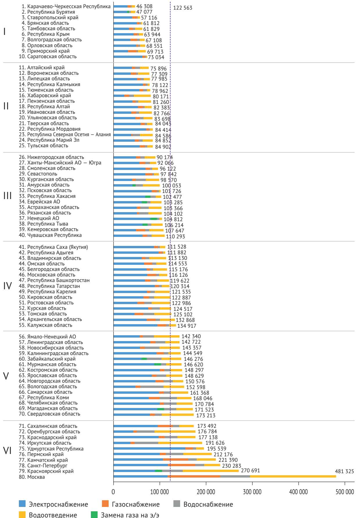
Рис. 90. Рэнкинг субъектов Российской Федерации по суммарной стоимости подключения с разделением по видам ресурсов в 2021 г., тыс. руб.
