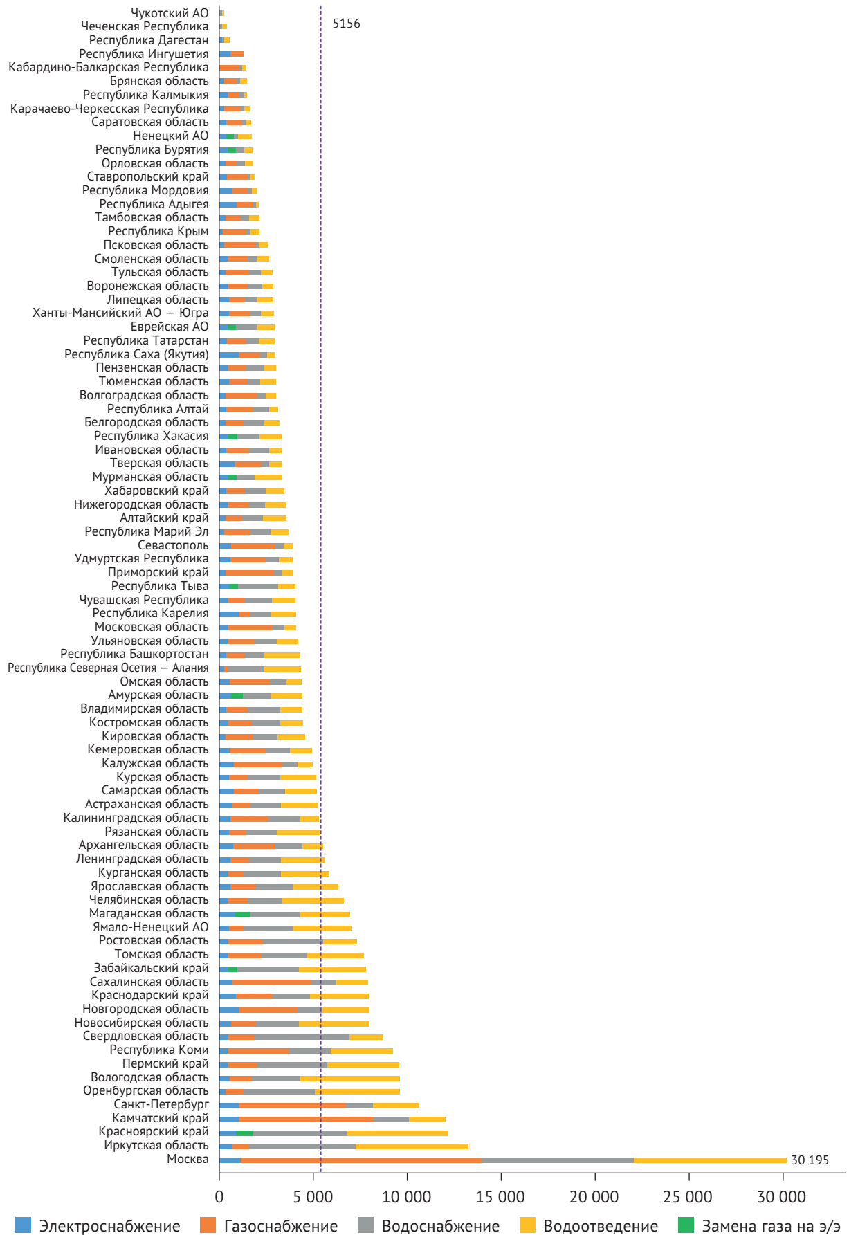
Рис. 72. Стоимость подключения кафе к сетям инженерно-технического обеспечения в 2021 г., тыс. руб.
