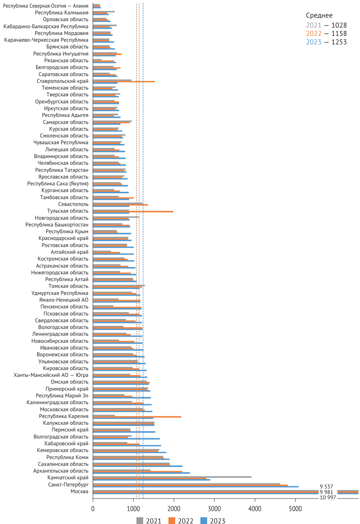
Рис. 36. Стоимость подключения коттеджа к сетям газораспределения, тыс. руб.
